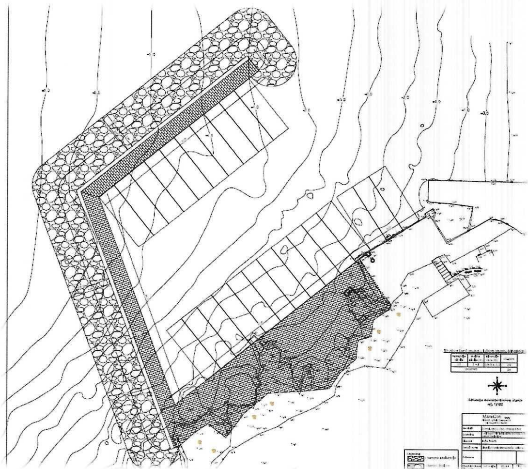
Izdvojeni lučki bazen luke Martinšćica - naselje Miholašćica
