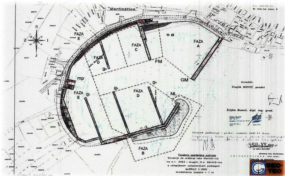
Rekonstrukcija-dogradnja luke otvorene za javni promet u naselju Martinšćica na otoku Cresu
