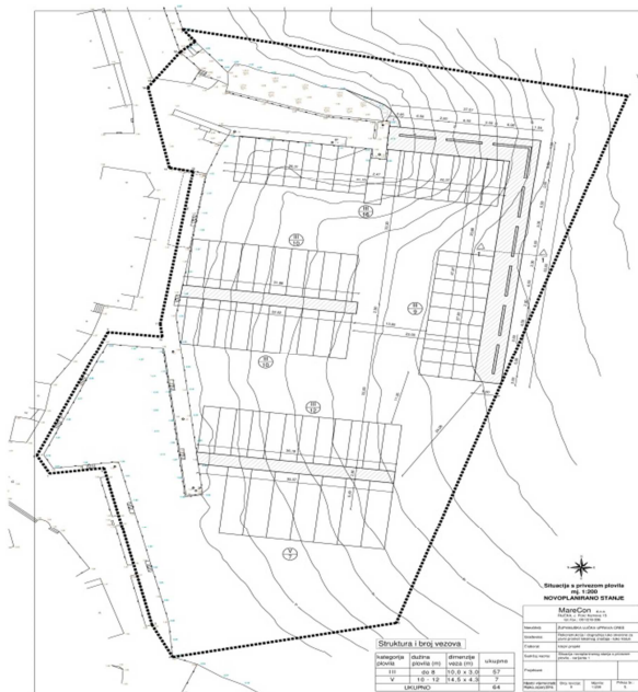
Idejno rješenje dogradnje luke Valun
