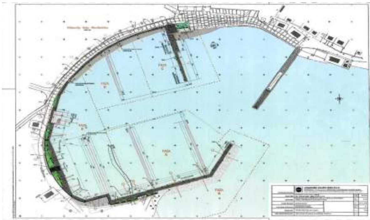
Rekonstrukcija – dogradnja luke otvorene za javni promet u naselju Martinšćica
